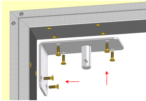
1. 상부힌지를 고정한다.(볼트, 용접, 피스)
