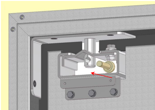
3. 상부축 홀에 롤러와 핀을 끼워 넣는다.
