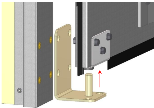
5. 하부힌지를 끼운다.(핀에 구리스 바름)
