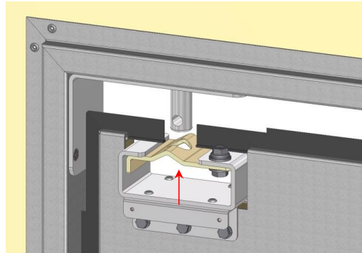
2. 도어를 상부축에 끼워 넣는다.
