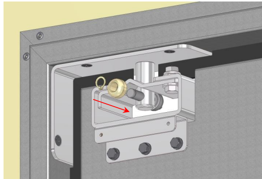
4. 반대편에 롤러와 스냅링을 끼운다.
