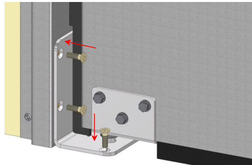
6. 하부힌지를 프레임과 바닥에 볼트와 앵커볼트로 고정한다.
