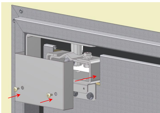
7. 롤러에 구리스를 바른 후 힌지커버를 닫는다.
